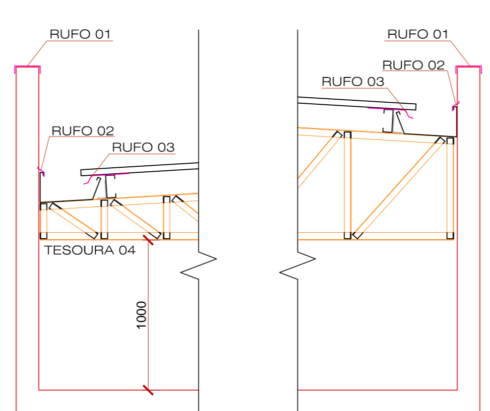
2 ESCALA 01 CORTE C-C SEM ESCALA
