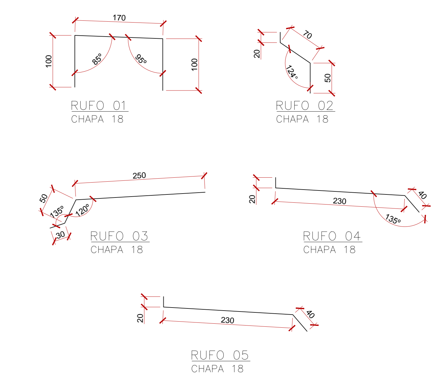
2 ESCALA 01 RUFOS SEM ESCALA
