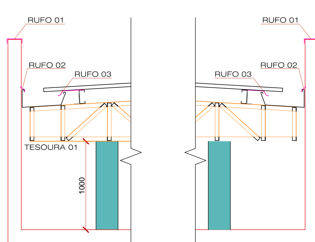
2 ESCALA 01 CORTE A-A SEM ESCALA
