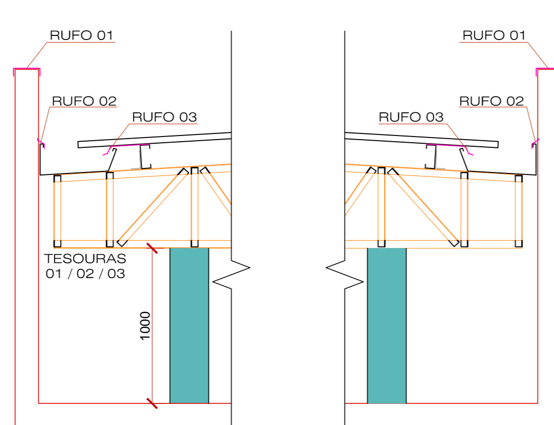
2 ESCALA 01 CORTE B-B SEM ESCALA
