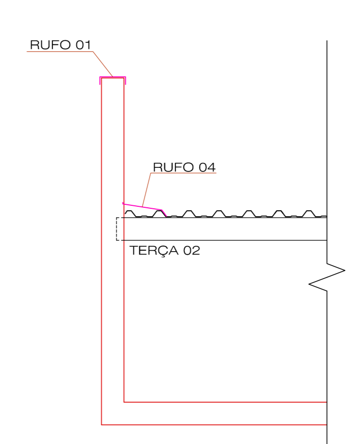
2 ESCALA 01 CORTE E-E SEM ESCALA
