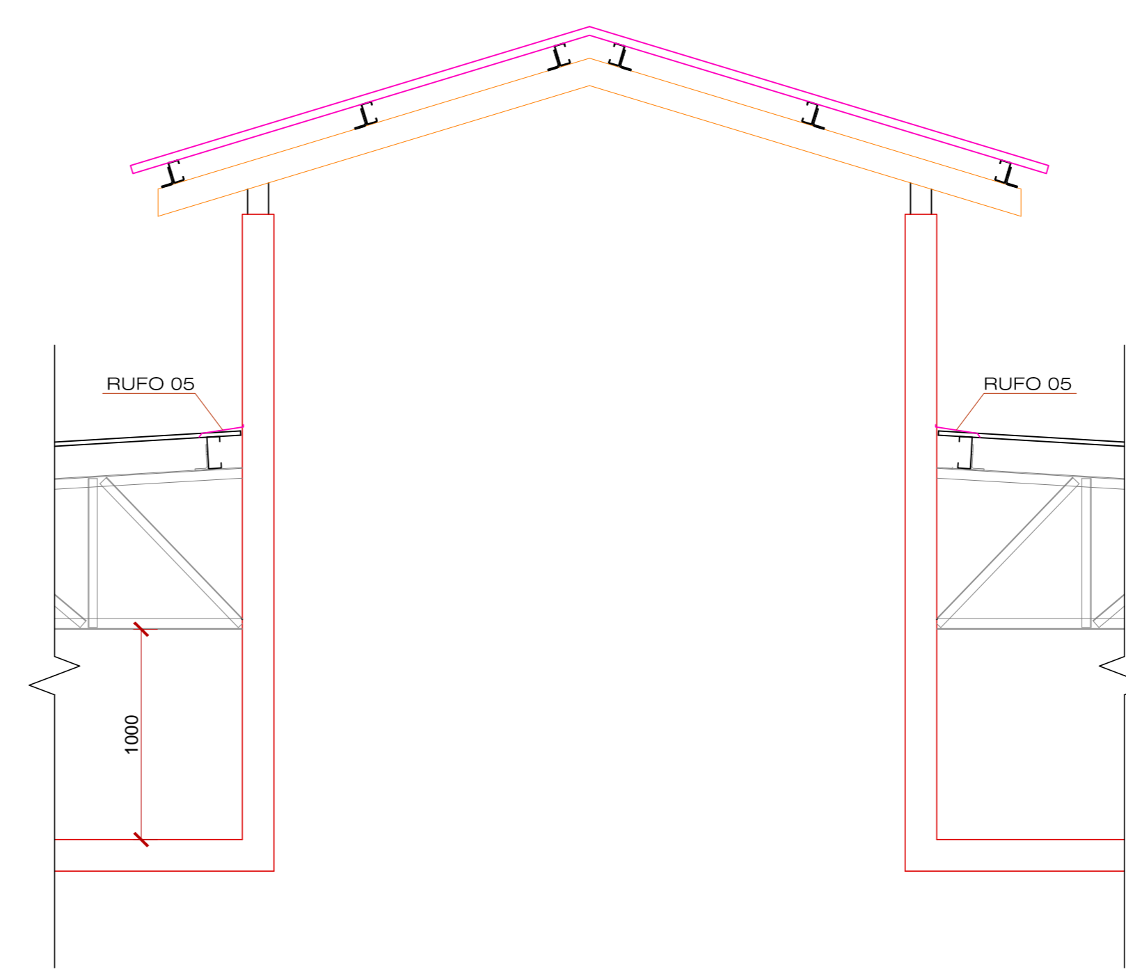
2 ESCALA 01 CORTE F-F SEM ESCALA
