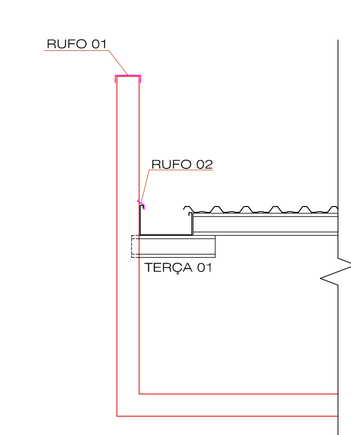
2 ESCALA 01 CORTE D-D SEM ESCALA
