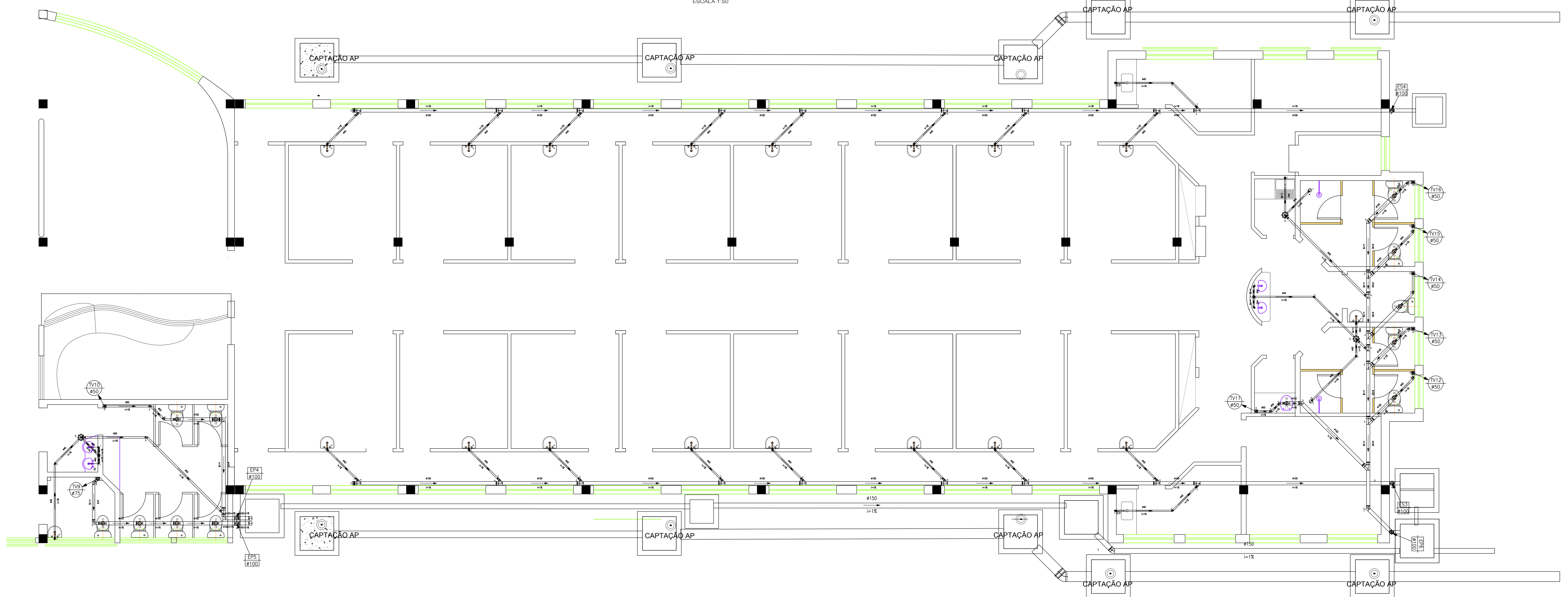
PLANTA - agua pluvial/esgotos ALA "A" - PAVIMENTO SUPERIOR ESCALA 1:50
