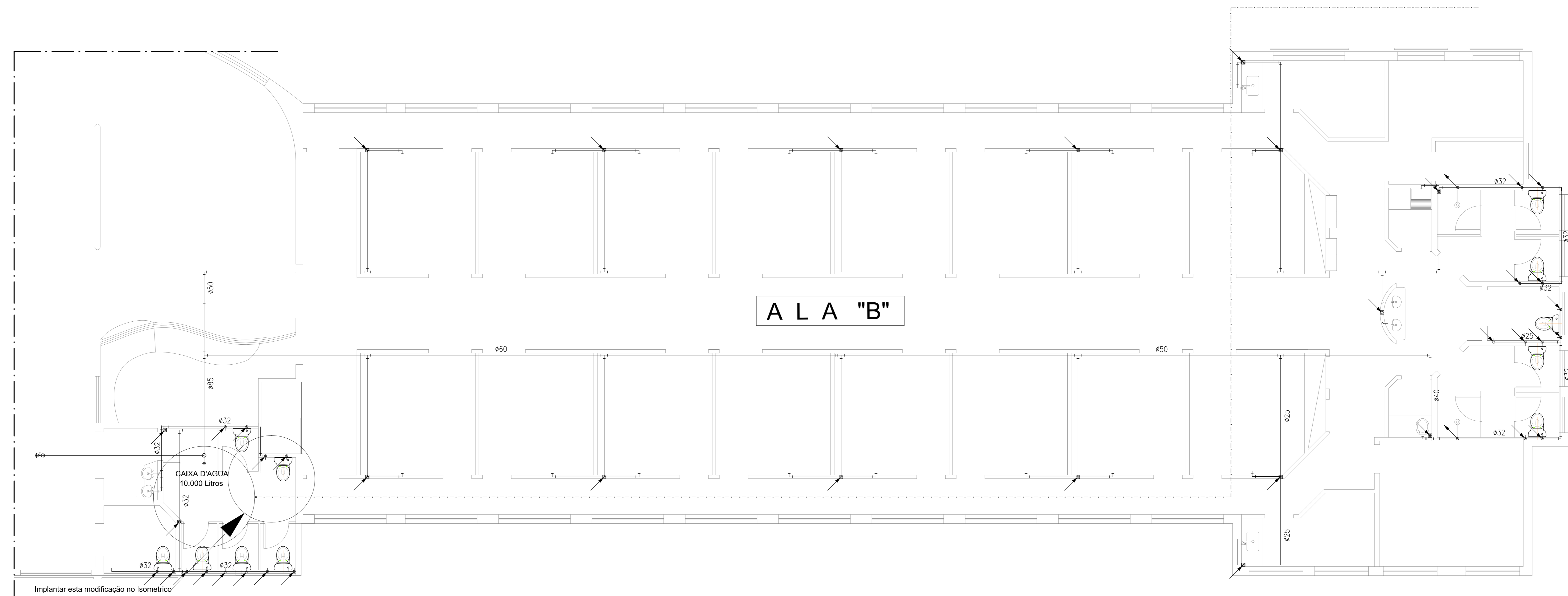
PLANTA - ÁGUA FRIA ALA "B" - PAVIMENTO SUPERIOR ESCALA 1:50
