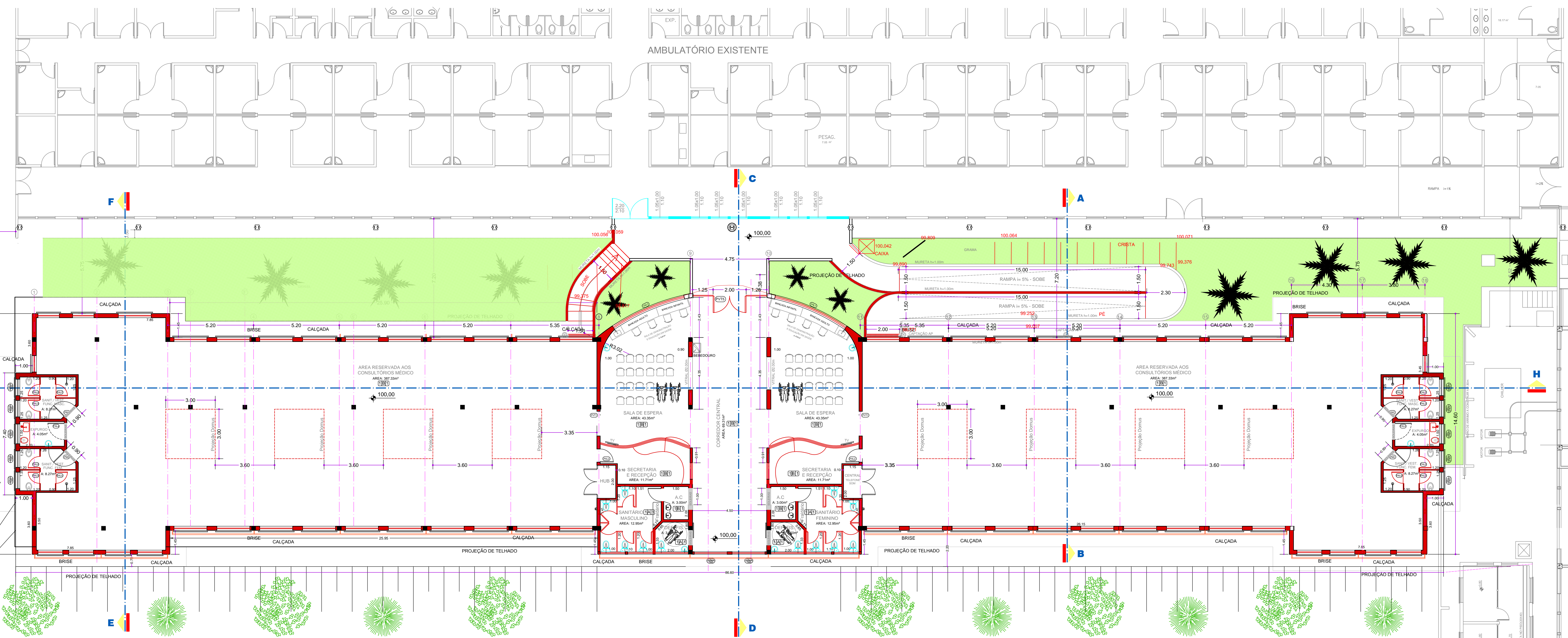
1 TOURS 02 PLANTA - AMBULATÓRIO PAVIMENTO TÉRREO ESCALA 1:100
