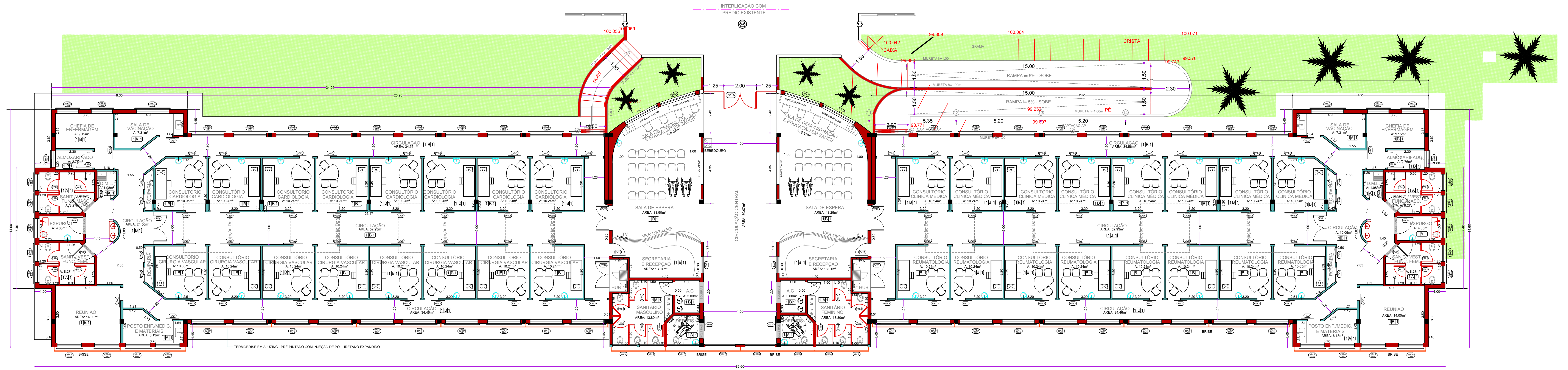
1 TOURS 02 PLANTA - AMBULATÓRIO PAVIMENTO TÉRREO ESCALA 1:100
